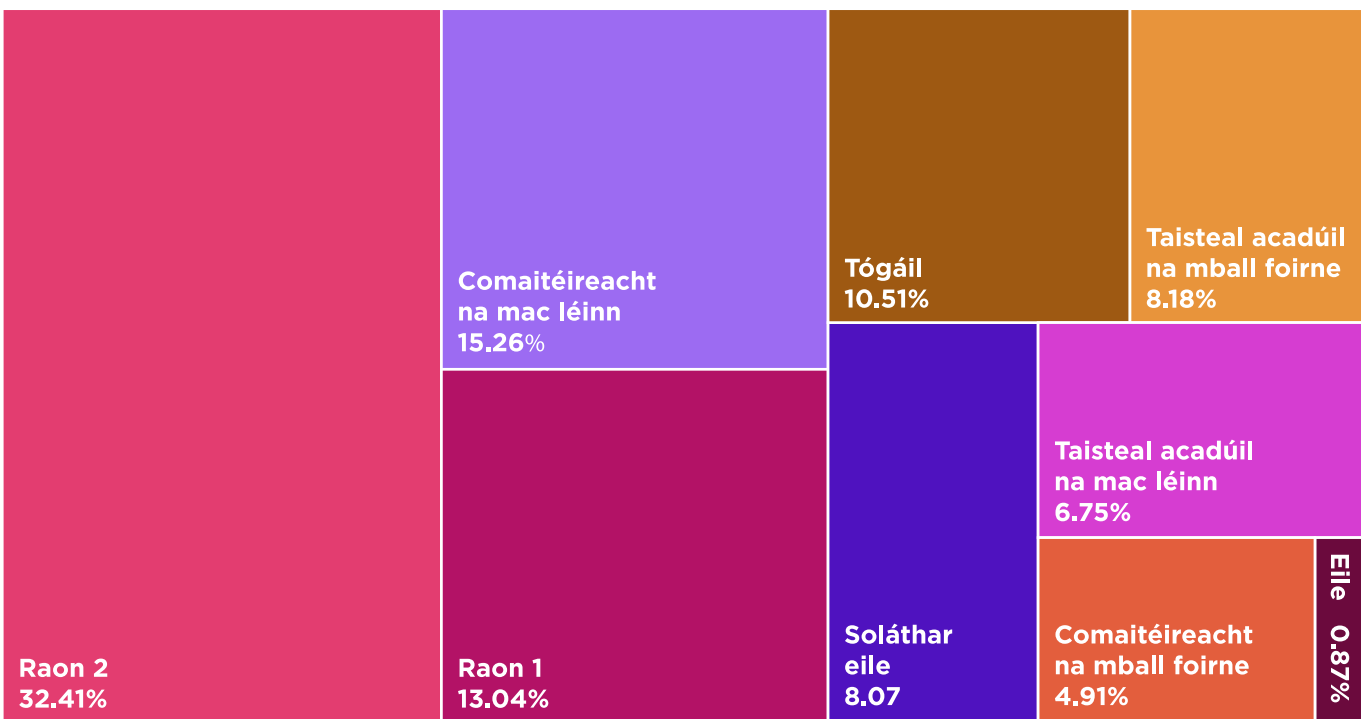
Fig 3. Miondealú lorg carbóin COC i gcatagóirí raon 1, 2 agus 3
