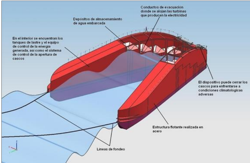
El esquema de funcionamiento del Wavecat muestra su estructura de catamarán. / VICUS
